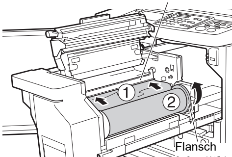
Masterführungslasche
